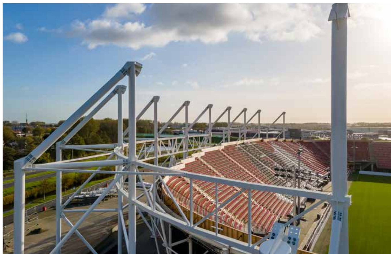
Buizen voor de nieuwe dakconstructie van het AZ Stadion.
